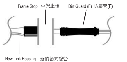
New Link Housing 新的節式線管
